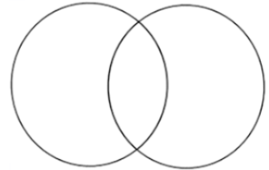
Venn diagram
