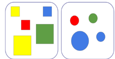
grouping
